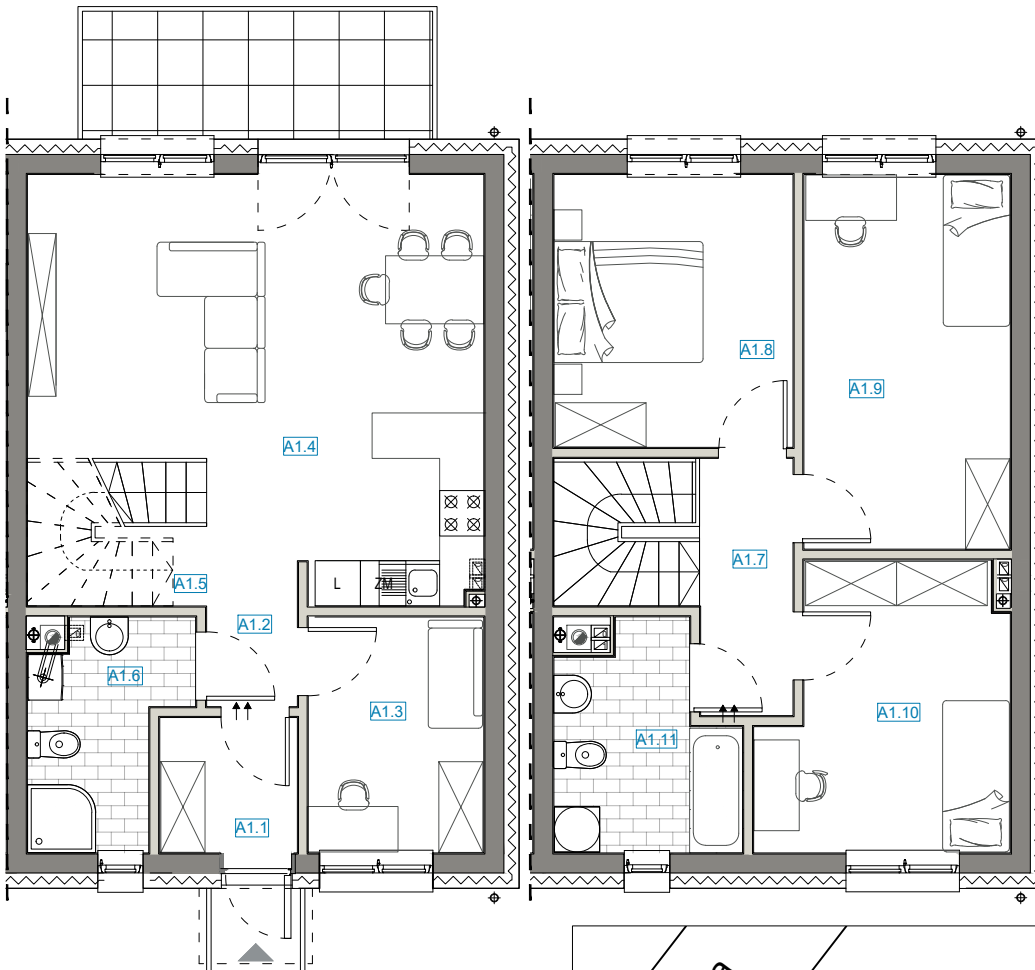
ZESTAWIENIE POWIERZCHNI POMIESZCZEŃ, PARTER, LOKALU A1
